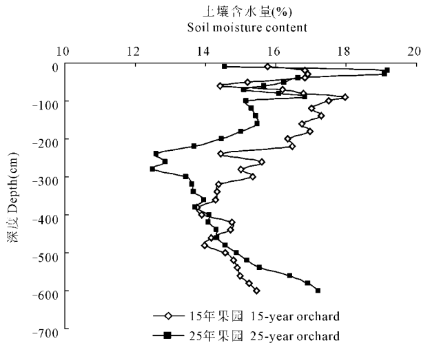
图2 不同果龄果园土壤水分分布
