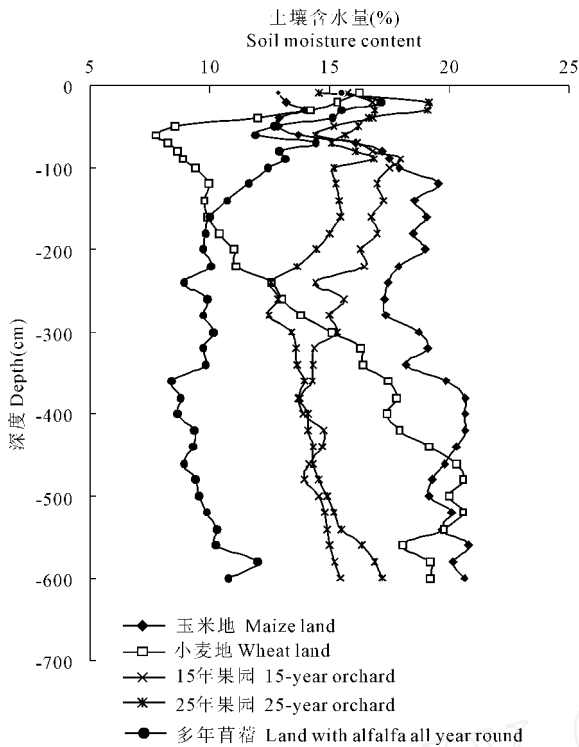
图 1 不同土地利用条件下的土壤水分分布
